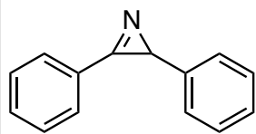
3 (CDCl 3 , 100 MHz)
